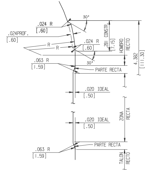
DETALLE DE PANEL ESCALA: 4=1
