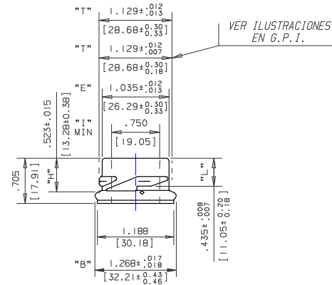
DETALLE DE ACABADO 30-2080-LA02 ESCALA: 1=1
